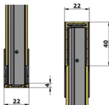
Sezione Verticale
