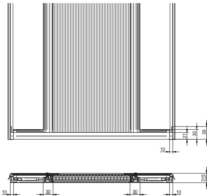
Sezione Orizzontale
