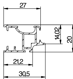
Sezione Barramaniglia
