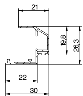
Sezione Guida
