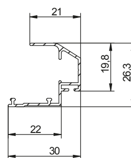
Sezione Guida
