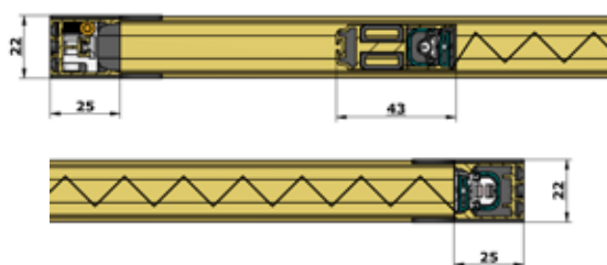
Sezione Orizzontale
