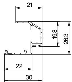
Sezione Guida
